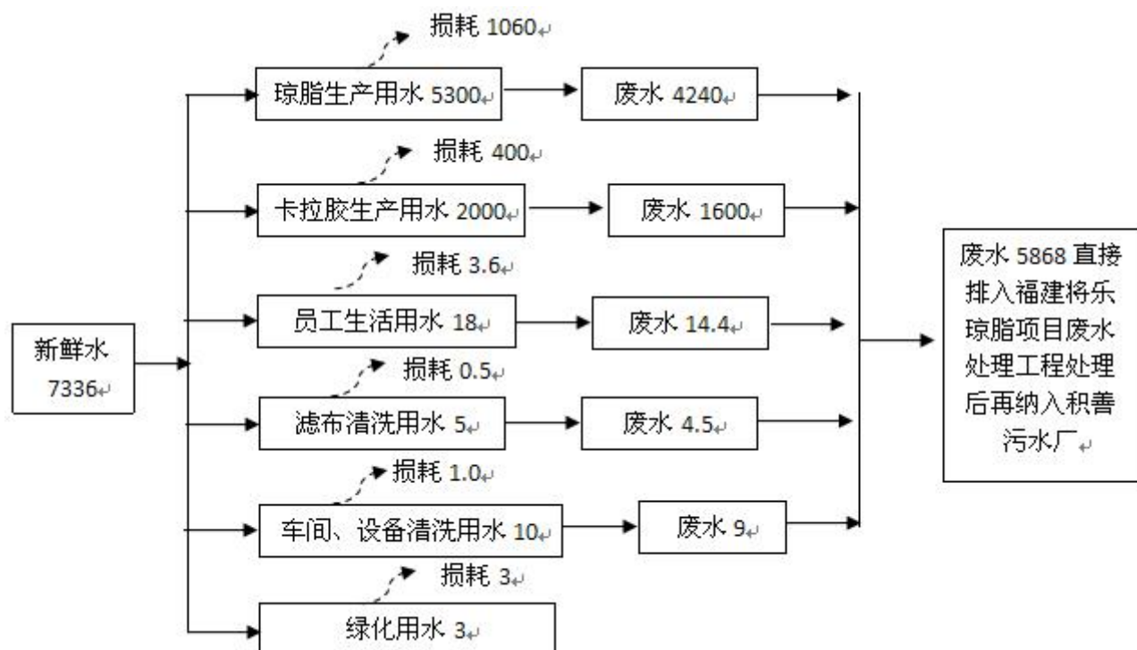
图 4.5-2 项目远期水平衡图 t/d
