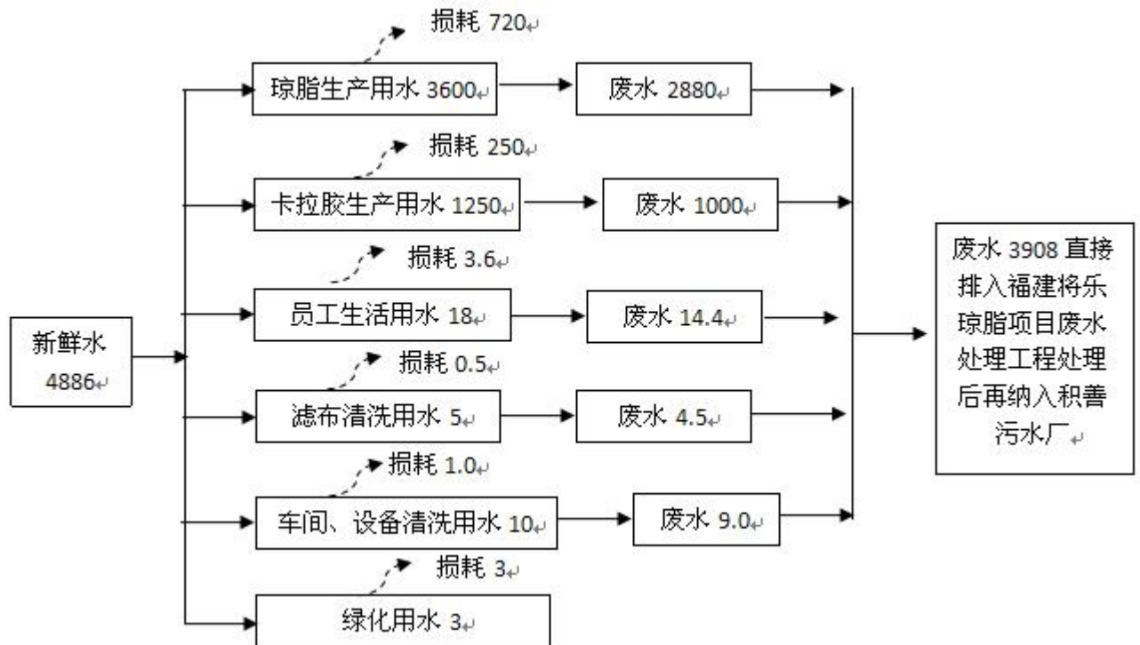
图 4.5-1 项目近期水平衡图 t/d
