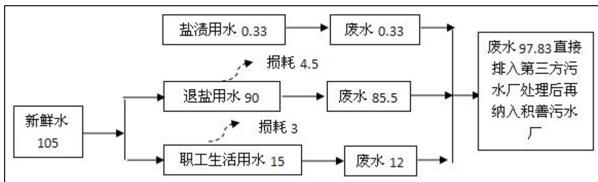
图 4.6-1 本项目用排水平衡 单位: t/d
