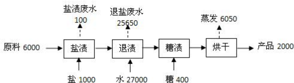
图 4.5-2 物料平衡图 单位：t/a
